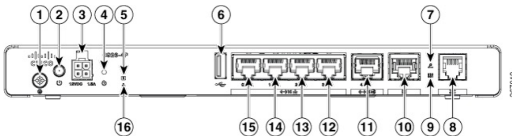
Abbildung 7: E/A-Ansicht des Cisco C926-4P
