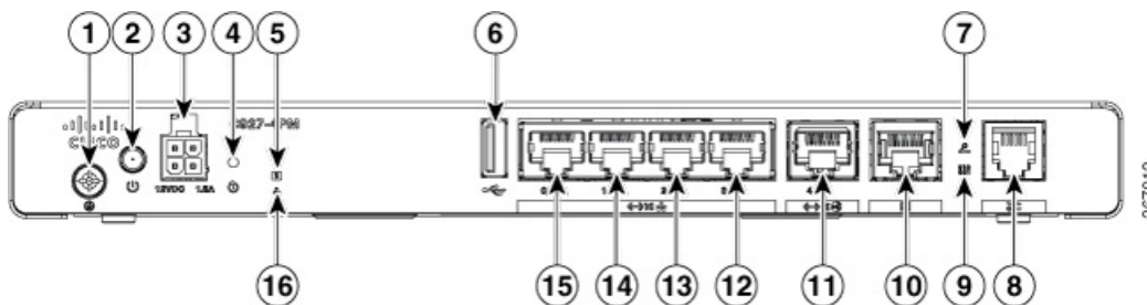
Abbildung 10: E/A-Ansicht des Cisco C927-4PM
