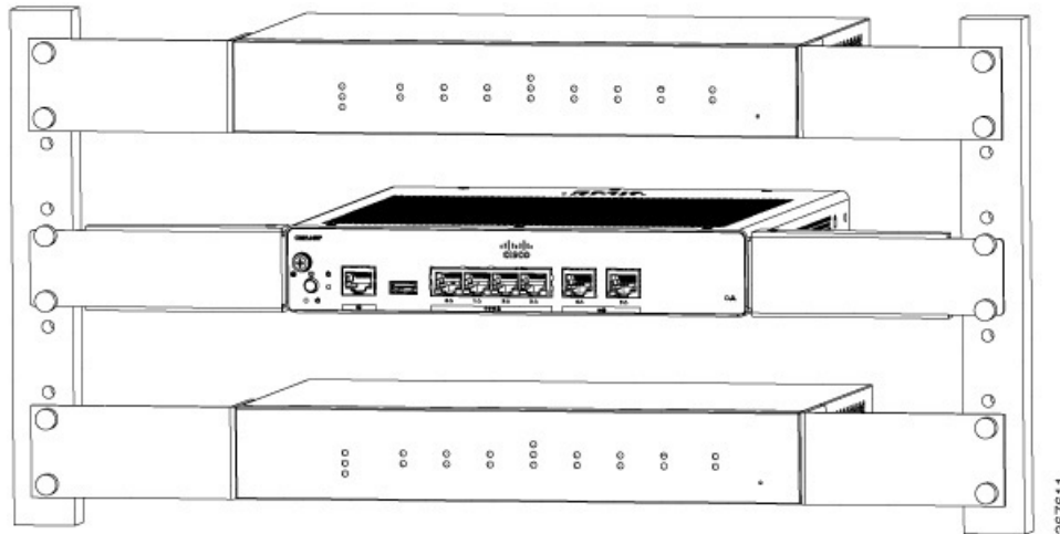
Abbildung 22: Montage der Cisco ISR-Router der Serie 900 in einem Rack
