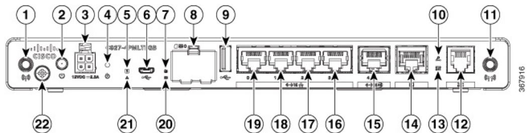
Abbildung 12: E/A-Ansicht des Cisco C927-4PMLTEGB
