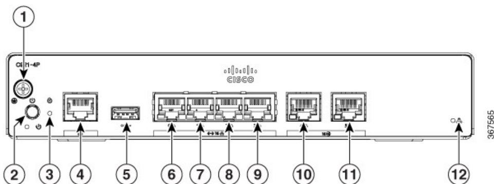
Abbildung 1: E/A-Ansicht des Cisco C921-4P
