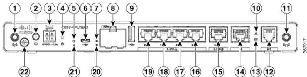
Abbildung 13: E/A-Ansicht des Cisco C927-4PLTEAU
