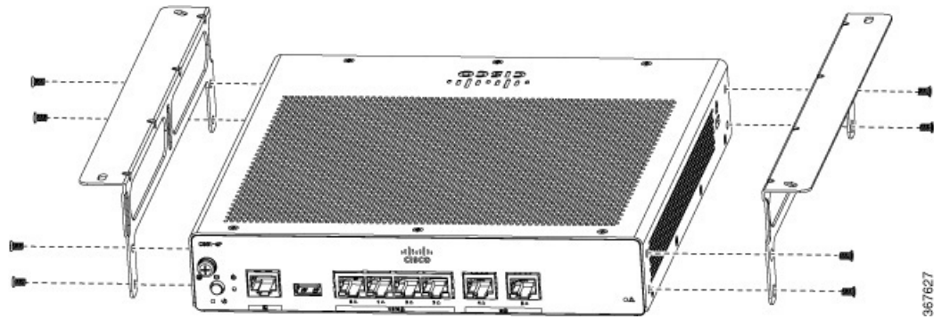
Abbildung 28: Flachkopfschrauben
