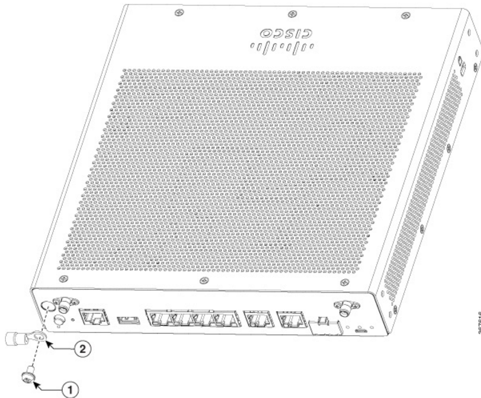
Abbildung 33: Chassis-Erdung – Cisco 900
