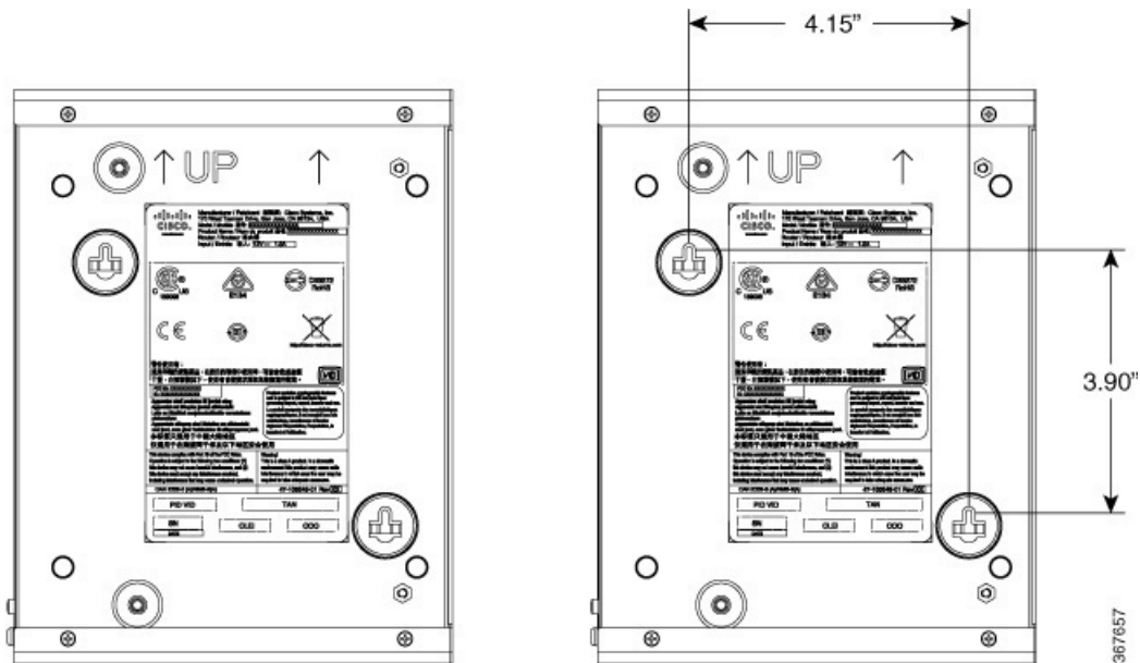
Abbildung 24: Router mit Wandmontagebohrungen auf der Unterseite
