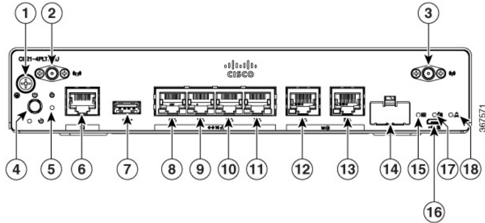
Abbildung 5: E/A-Ansicht des Cisco C921-4PLTEAU
