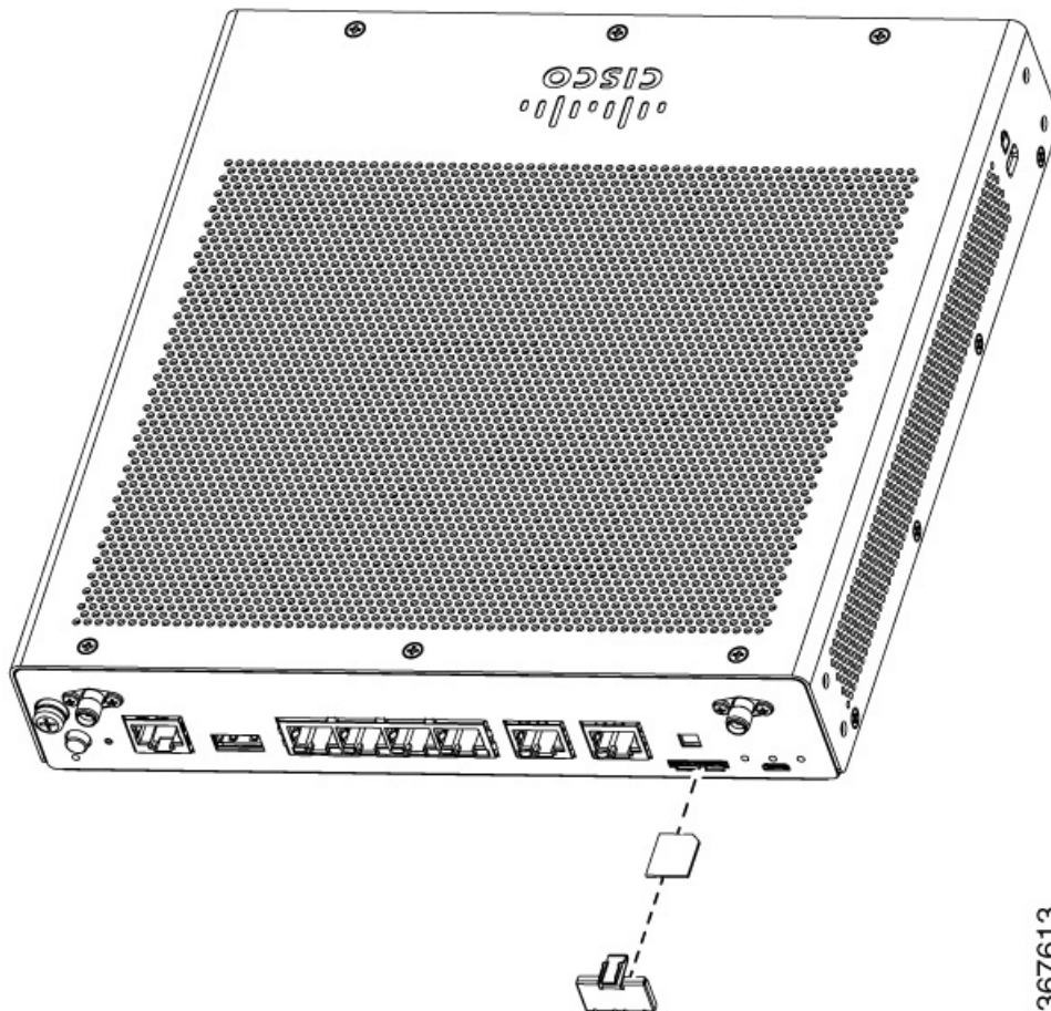
Abbildung 32: Einlegen der SIM-Karte
