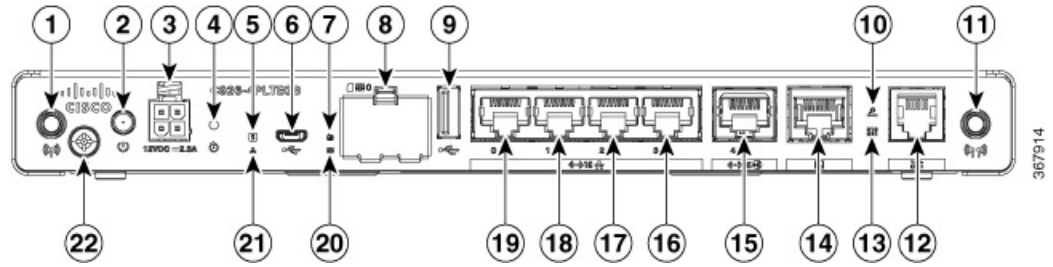
Abbildung 8: E/A-Ansicht des Cisco C926-4PLTEGB
