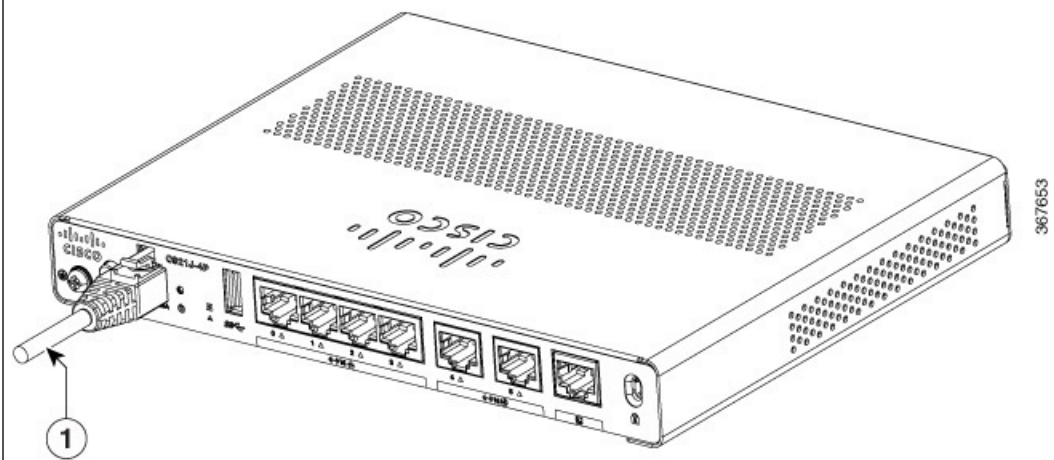
Abbildung 35: Router mit externem Netzteil
