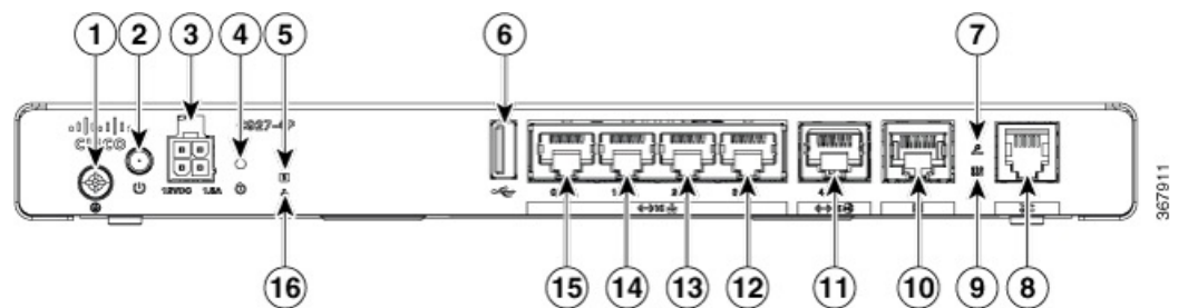
Abbildung 9: E/A-Ansicht des Cisco C927-4P
