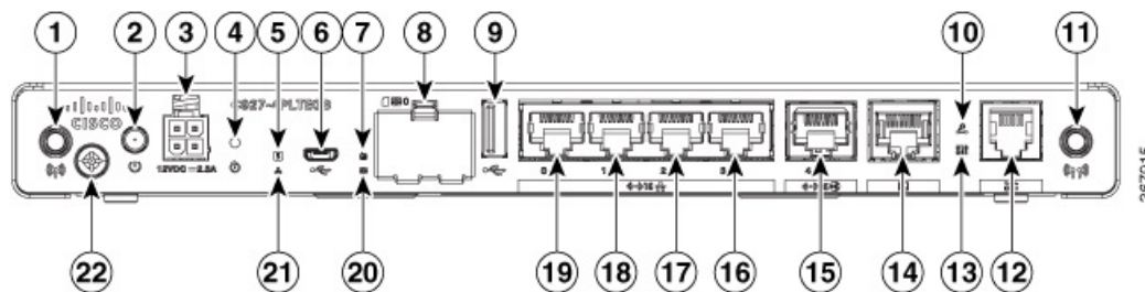
Abbildung 11: E/A-Ansicht des Cisco C927-4PLTEGB
