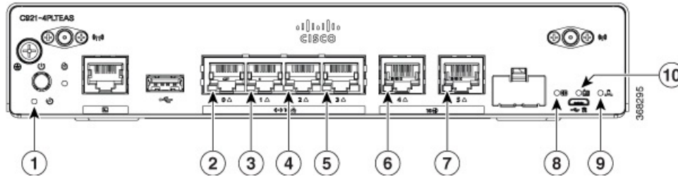
Abbildung 17: LED-Kontrollleuchten an 4G-LTE-SKUs – E/A-Seite
