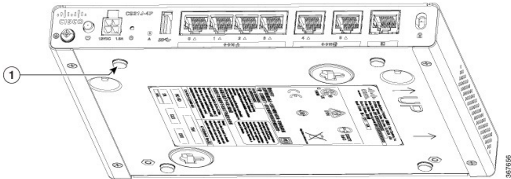
Abbildung 26: Unterseite des Routers mit Gummifüßen
