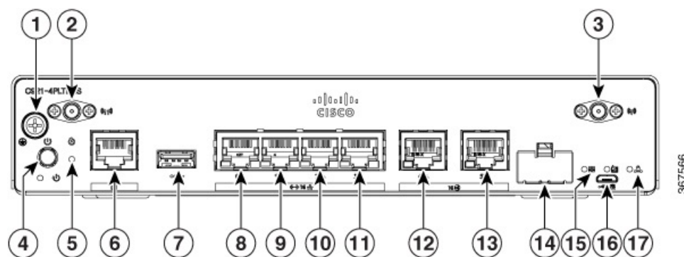
Abbildung 3: E/A-Ansicht des Cisco C921-4PLTENA
