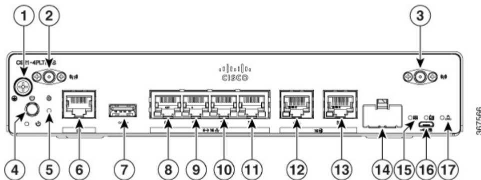
Abbildung 4: E/A-Ansicht des Cisco C921-4PLTEAS
