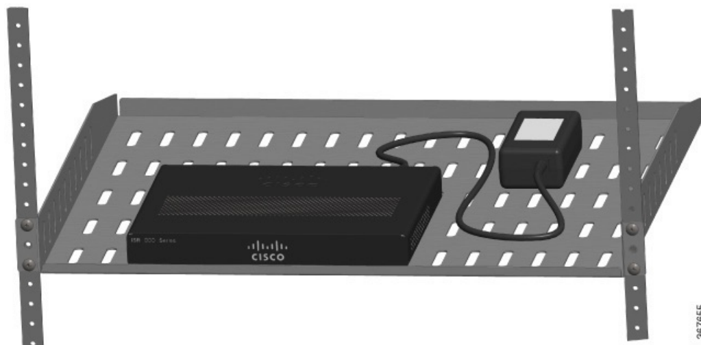
Abbildung 23: Montage der Cisco ISR-Router der Serie 900 in einem Einschub
