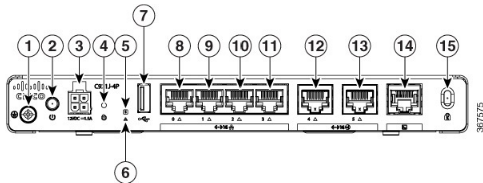
Abbildung 2: E/A-Ansicht des Cisco C921J-4P
