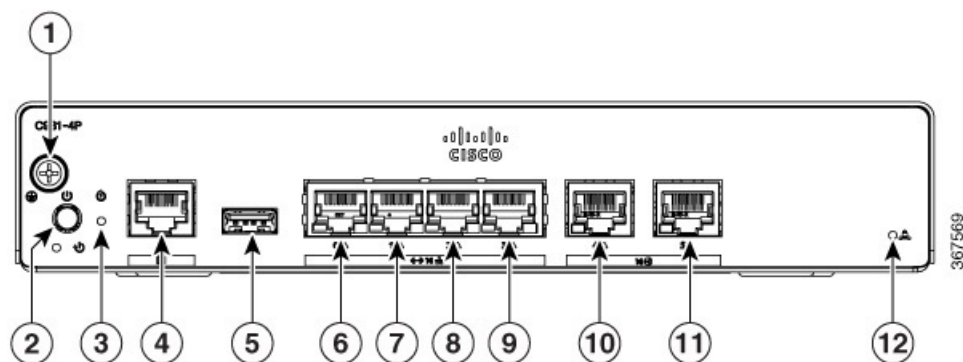
Abbildung 14: E/A-Ansicht des Cisco C931-4P
