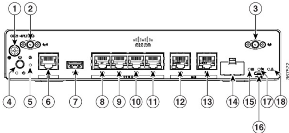
Abbildung 6: E/A-Ansicht des Cisco C921-4PLTEGB
